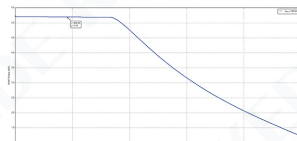
电机TN图 Motor TN diagram
